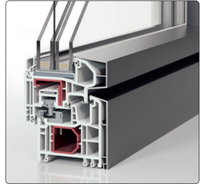
PaXabsolut Alublend flächenbündig
