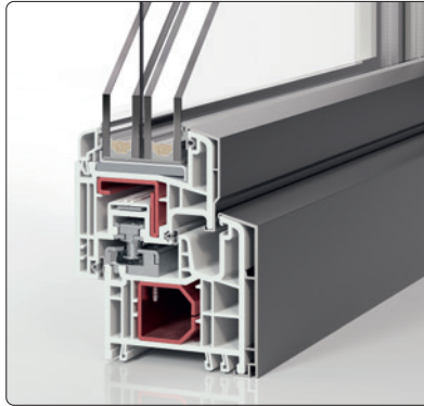
PaXabsolut Alublend flächenversetzt
