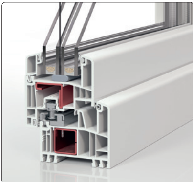
PaXabsolut Neo flächenversetzt
