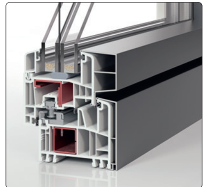
PaXabsolut Neo Alublend flächenbündig
