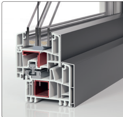
PaXabsolut Neo Alublend flächenversetzt
